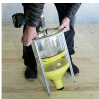
Placer l'aide au remplissage EASY FILL sur l'ouverture de la CLT BOX – DECKE FS
