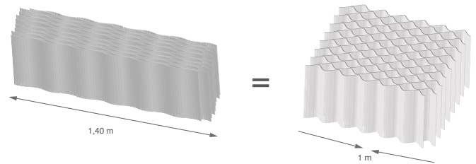
La largeur est réduite quand les alvéoles sont étirées / Width is reduced when the cells are stretched
